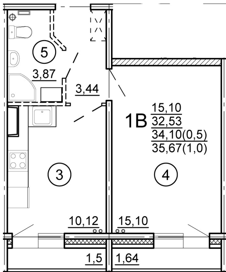
План этажа:
